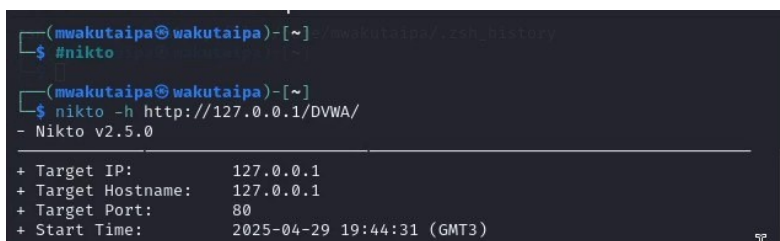
Рис. 3: Сканирование 1 с nikto
